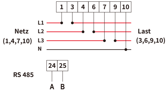
Abb. 7.9 CHINT-Zähler
