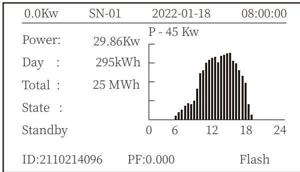
Abb. 8.1 Die Ausgangsschnittstelle
