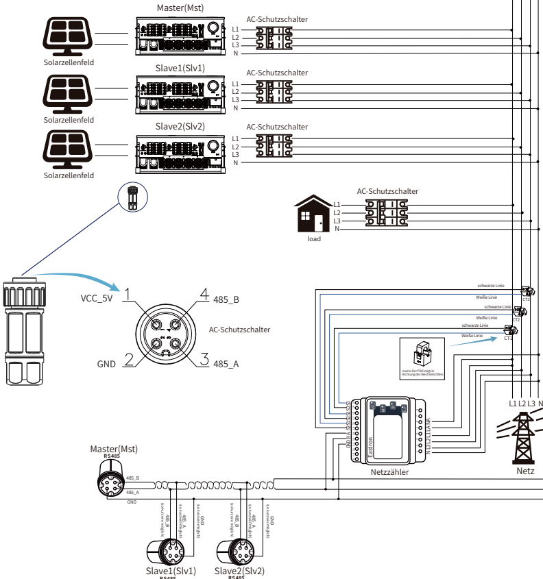
Abb. 7.25 Anschlussplan (Dreiphasenstrom)
