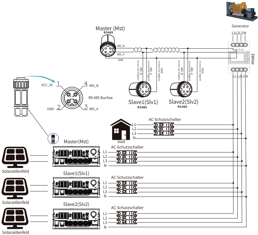
Abb. 7.23 EASTRON Anschlussplan (Die Durchleitungstabelle)
