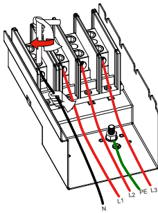
Abb. 5.9 AC-Kabel an die Klemme angeschlossen
