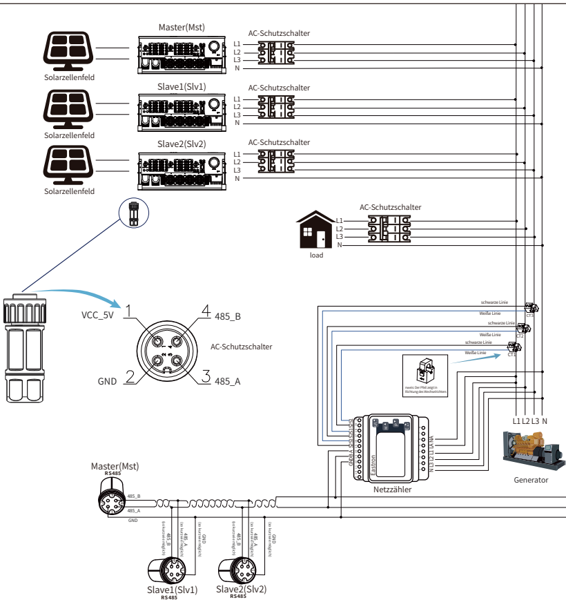
Abb. 7.27 Anschlussplan (Dreiphasenstrom)
